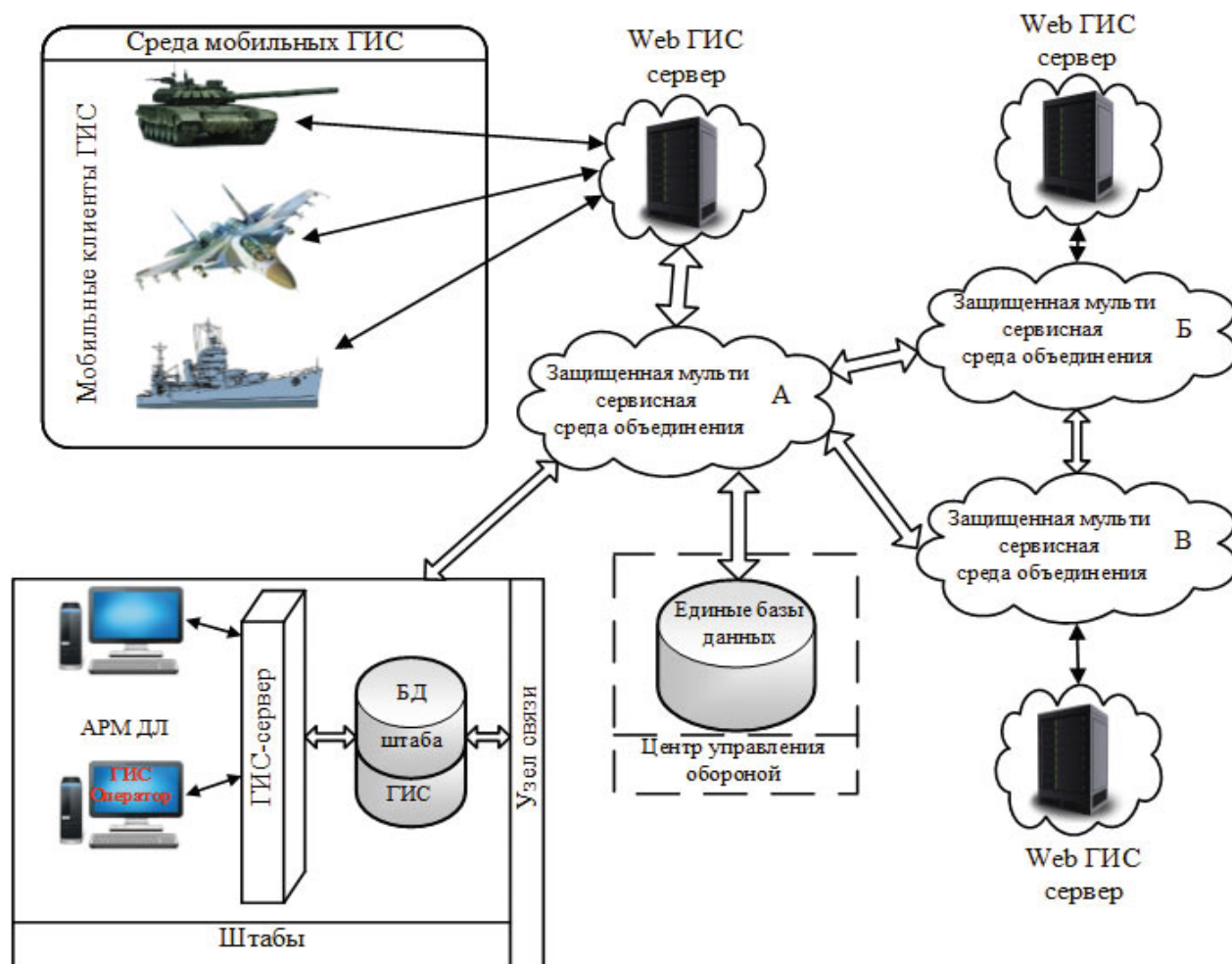
Рисунок 1 – Структура узла сетевцентрической системы управления
