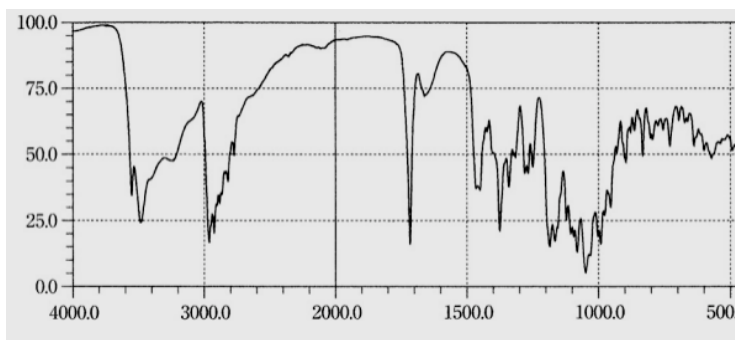
Рисунок 3 – ИК-спектр стандарта Азитромицина
