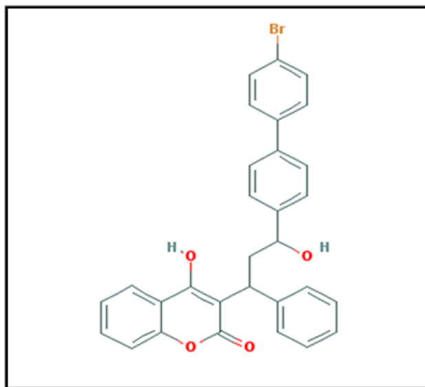
Рисунок 1 – Структура бромадиолона
