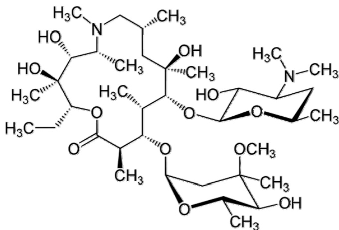
Рисунок 1 – Структурная формула азитромицина
