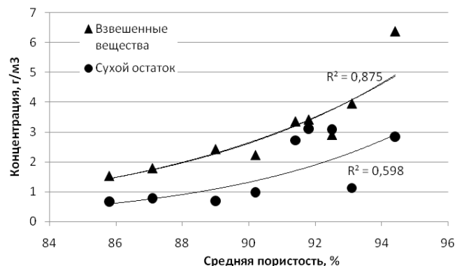
Рис. 1. Зависимость количества взвешенных веществ и сухого остатка от пористости снежного покрова
