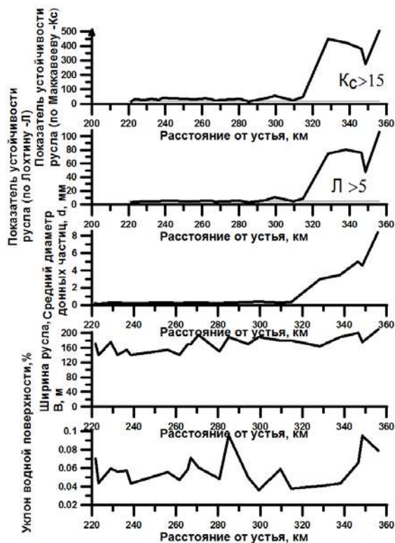
Рис. 1. Изменения русловых характеристик и показателей устойчивости к размыву р. Днестр на участке г. Дубоссары – г. Бендеры
