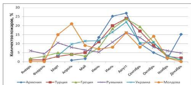
Рис. 2. Сезонная (а) и годовая (б) повторяемость пожаров в странах-партнерах проекта (Zibtev et al., 2013)
