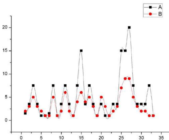
Рис. 2. Связь между реальным темпом эрозии (А), т/га в год и полученным в результате моделирования по RUSLE 2 (В), т/га в год
