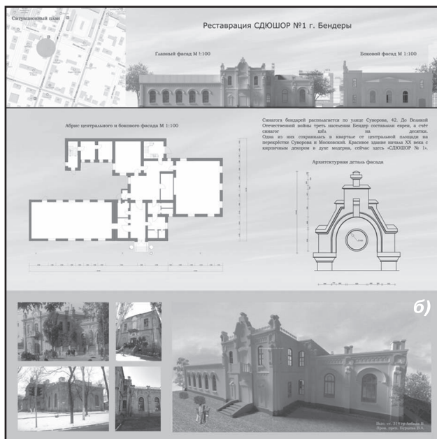
Фото 2. а, б) проект реставрации здания синагоги бондарей в г. Бендеры. Выполнен студенткой III курса кафедры архитектуры и дизайна БПФ ПГУ Лобода В.А.
